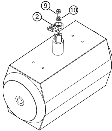
图 4-3 传动销
