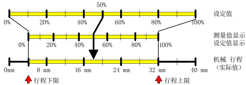
图 8-3 示例: YNRM = FLoW, YA = 10 %, YE = 80 %
