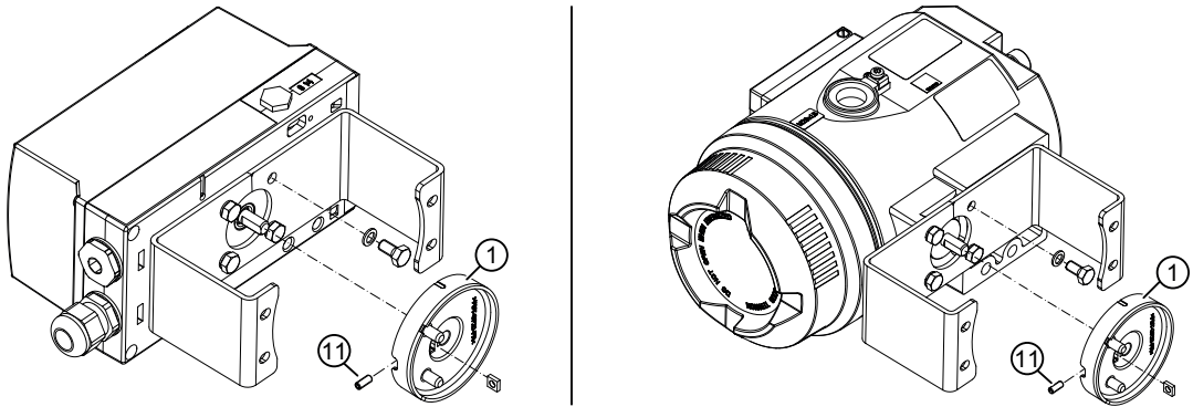
图 4-2 左侧：耦合轮，右侧：耦合轮，隔爆外壳
