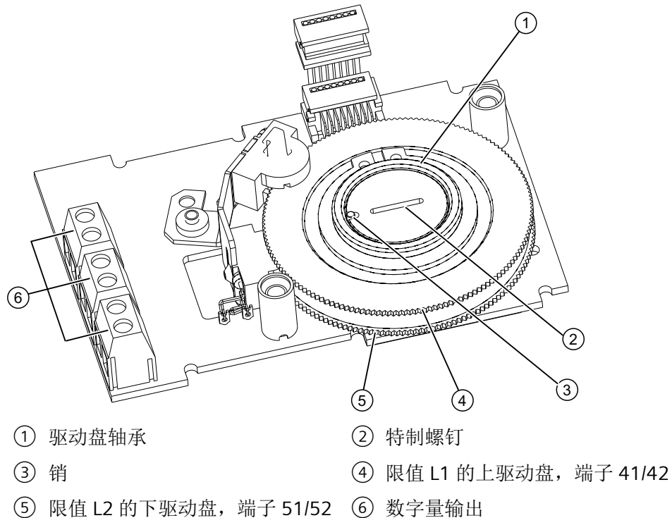
图 4-12 Inductive Limit Switches (ILS)，示意图
