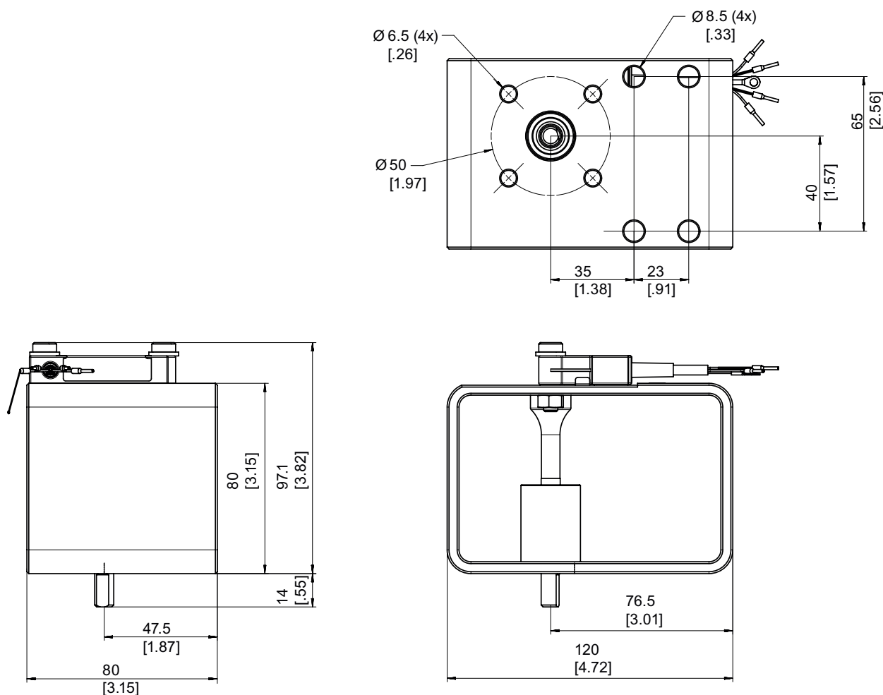
图 A-9 大于 14 mm (0.55 英寸) 的 NCS 模块尺寸图
