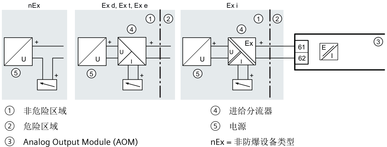
图 5-7 Analog Output Module (AOM)
