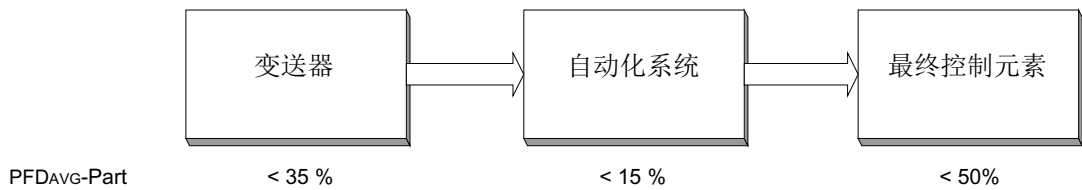
图 9-3 PFD 分布
