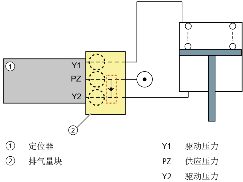
图 17-1 排气量块的工作模式
