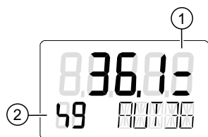
图 8-5 用两列显示阈值 2 错误消息（要求维护）
