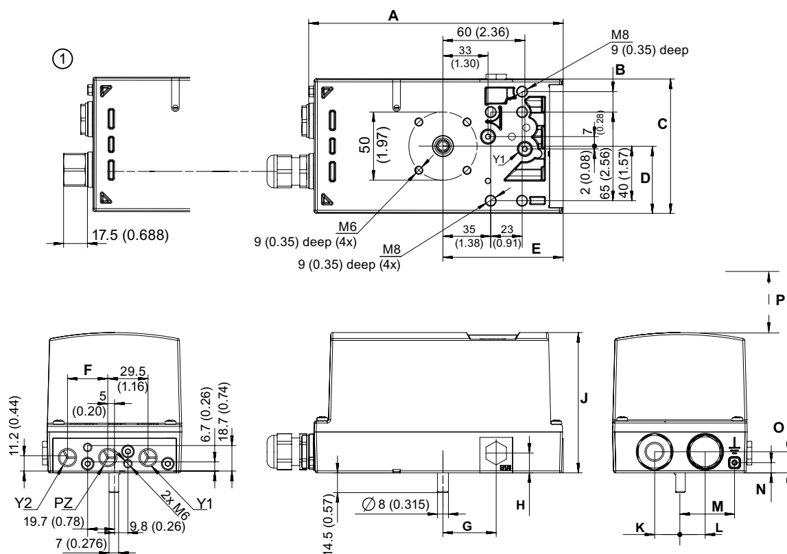
图 14-1 尺寸图，单位为 mm（英寸）
