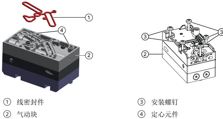
图 11-1 气动块
