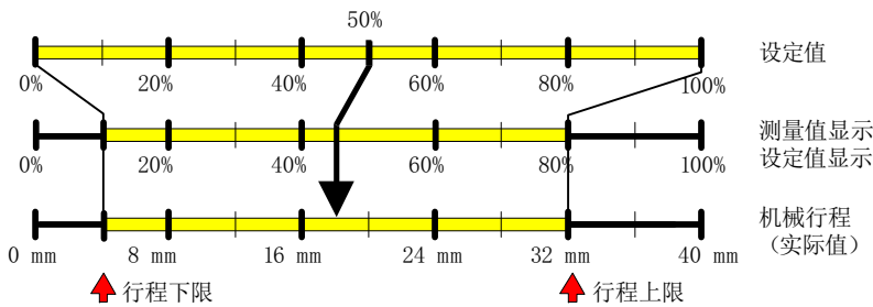
图 8-1 YNRM = MPOS 或 YNRM = FLoW; 默认: YA = 0 % 和 YE = 100 %
