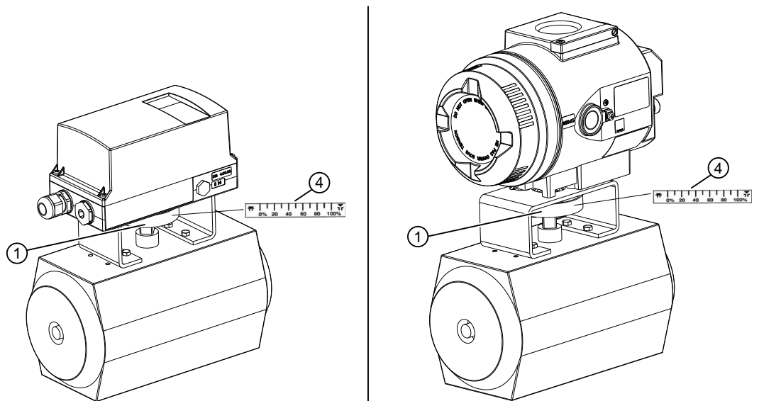
图 4-5 左侧：带刻度的不干胶标签；右侧：带刻度的不干胶标签，隔爆外壳
