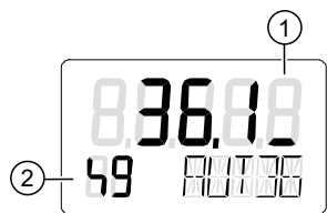
图 8-4 用一列显示阈值 1 错误消息（需要维护）
