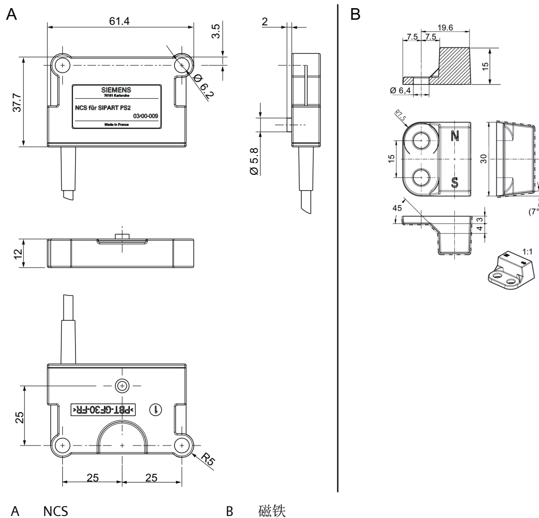
图 A-8 NCS 和磁铁的尺寸图
